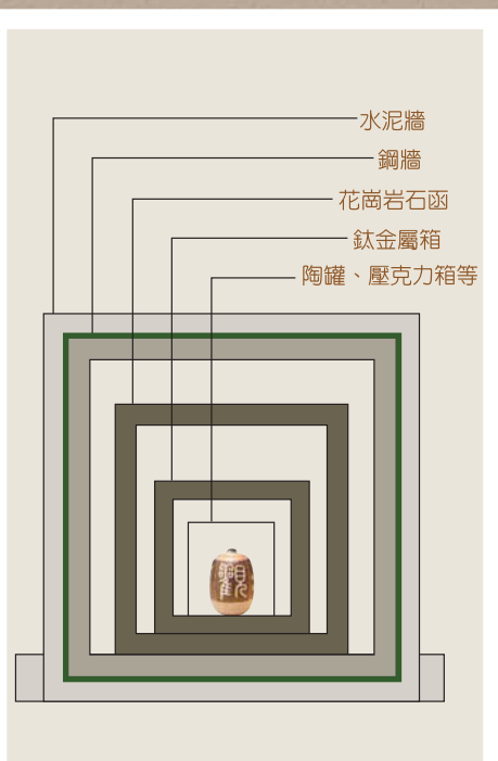
地宮構造剖面圖
